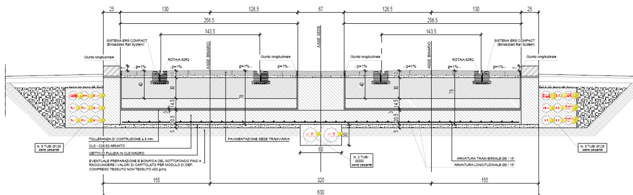
SEZIONE TRASVERSALE SEDE A DOPPIO BINARIO CON MATERASSINO - Scala 1:20
