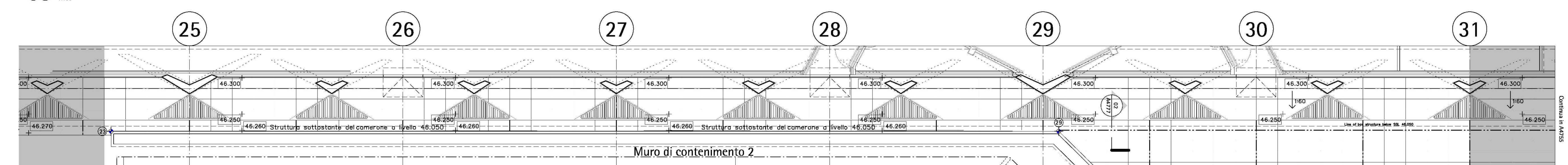
04 Pianta 1:100
