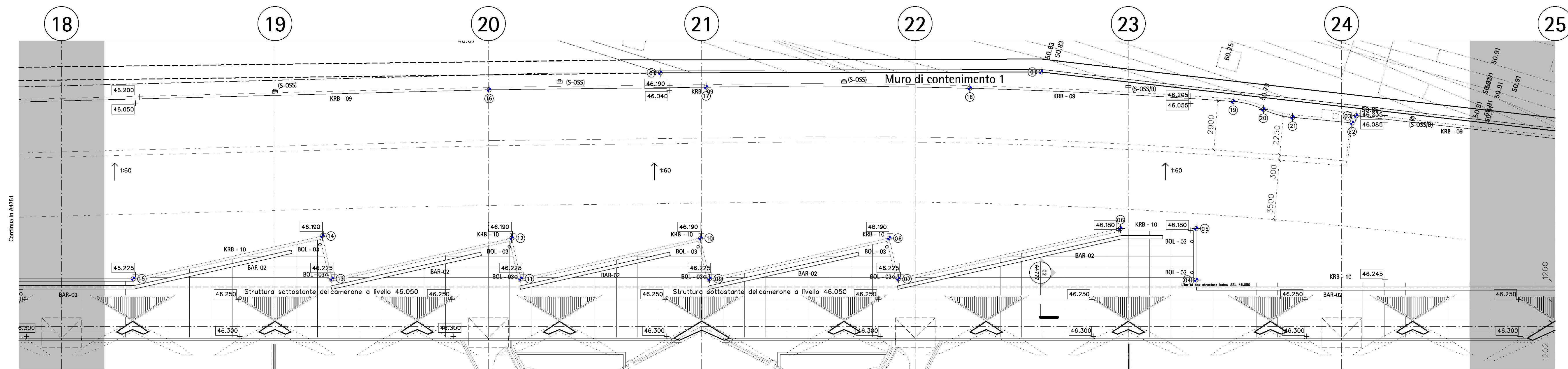
01 Pianta 1:100
