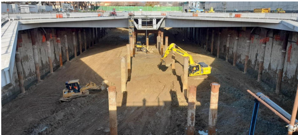
Foto 01 – attività di scavo all'interno del Camerone della Nuova Stazione AV
